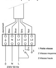
Schéma de principe RS 3
